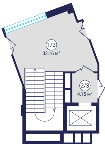
План 3-го поверху
