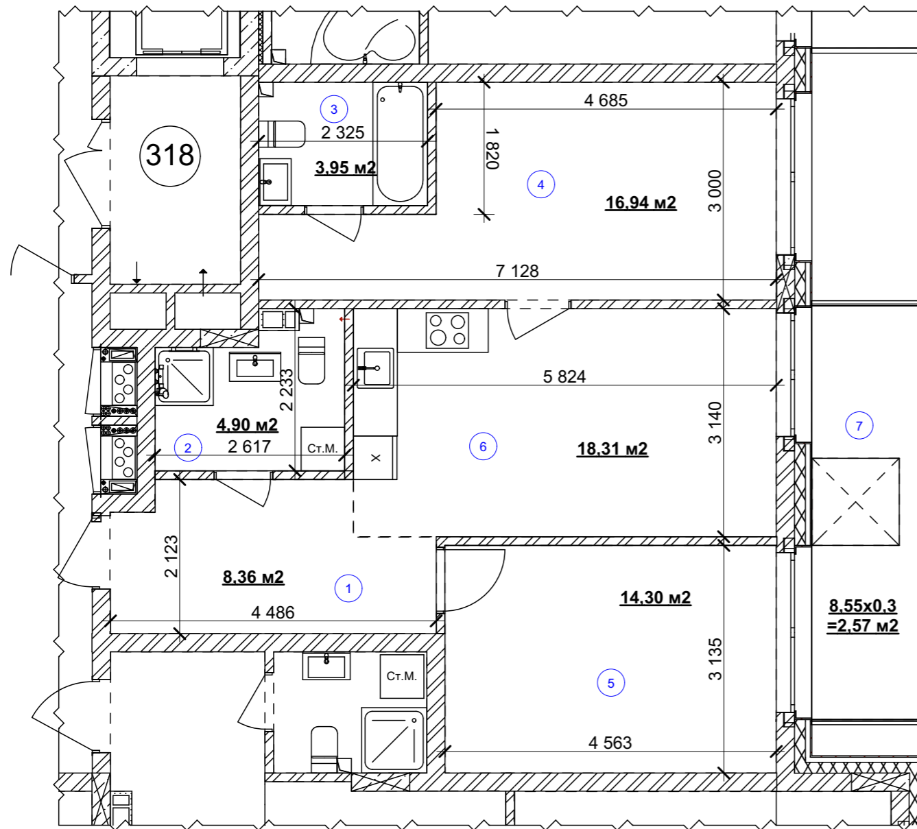
План 2 кімнатної квартири №82
