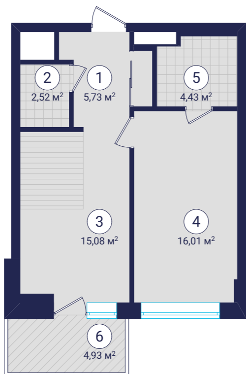
План 1-кімнатної квартири №104
